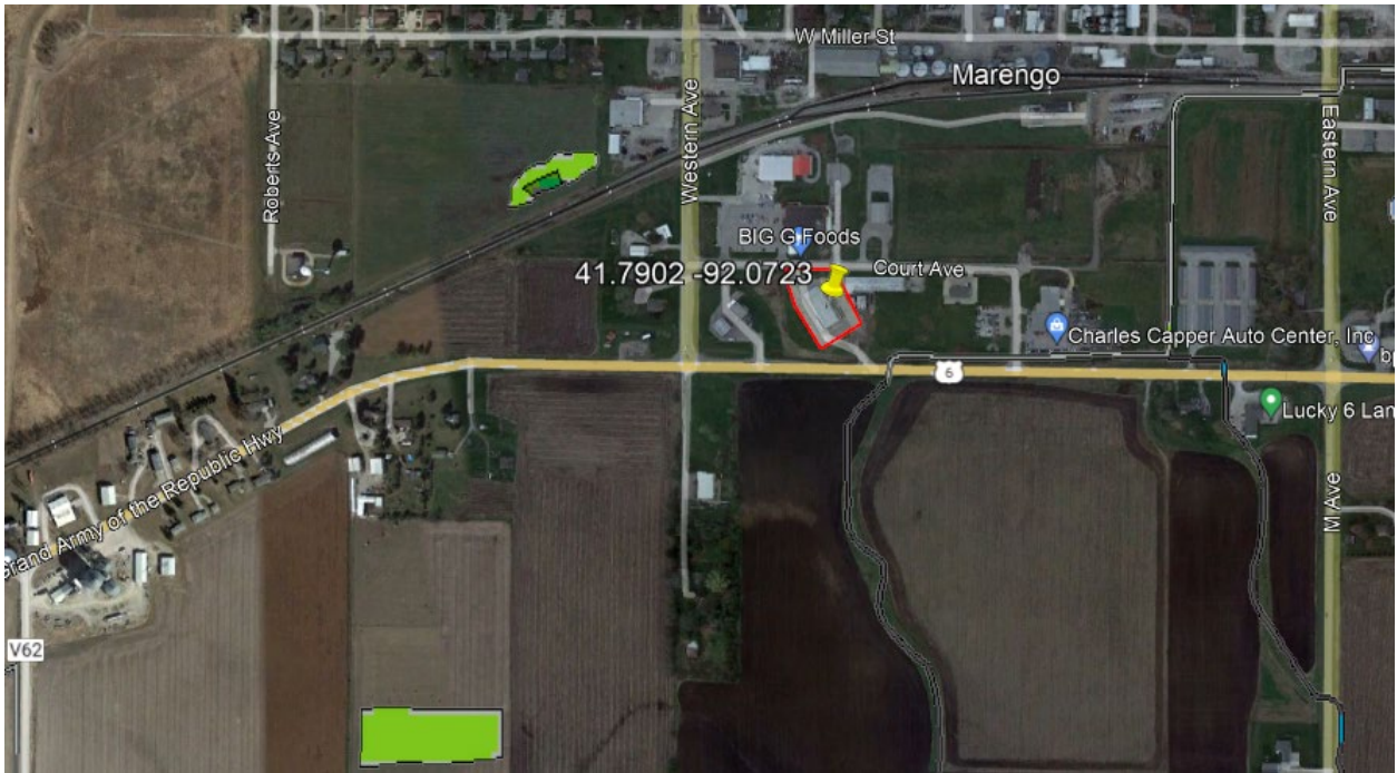
USFWS NWI
